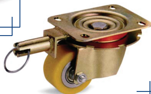
Ролик с фиксацией в 4-х или 8-ми положениях для театральных декораций.
